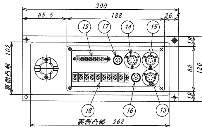
裏側端子部詳細
