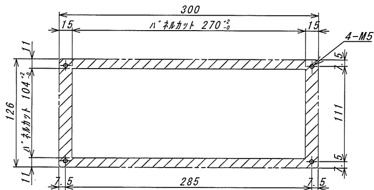
パネルカット寸法
