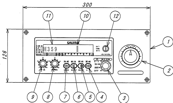
前面操作パネル詳細
